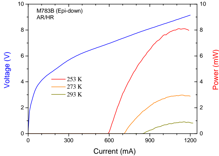
CW L-I-V Characteristics
